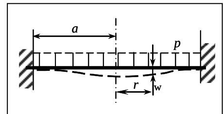
Fig.1 等分布荷重を受ける円板
