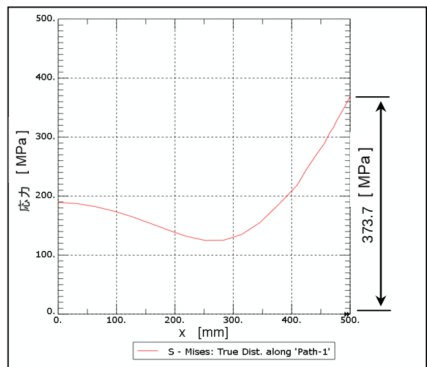
Fig.5 相当応力
