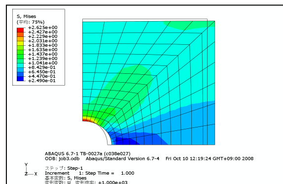
Fig.2 ミゼス応力分布
