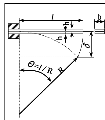
Fig.1 バイメタル
