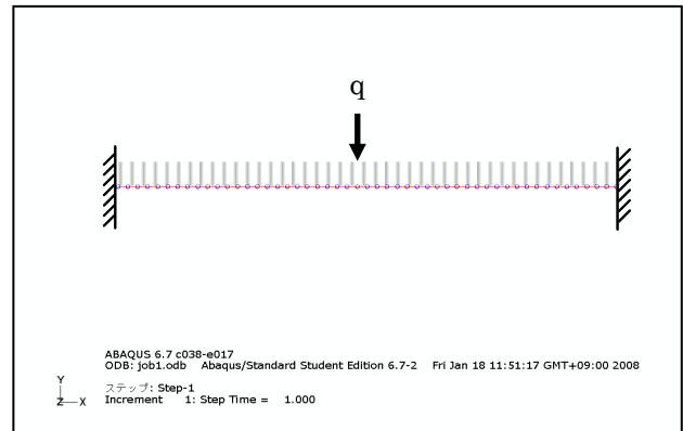
Fig.3 解析モデル
