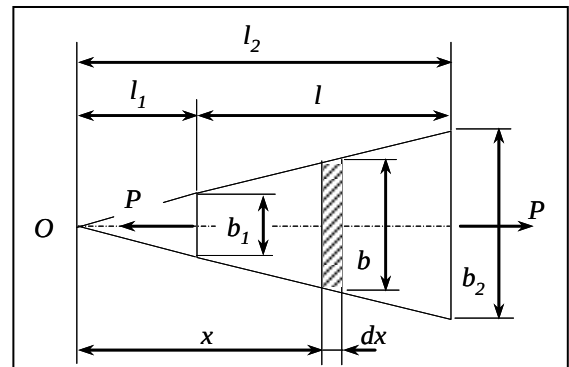
Fig.1 引張荷重を受ける台形板
